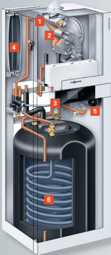
Vitodens 222-F mit emailiertem Rohrwendel-Warmwasserspeicher für Gebiete mit hartem Wasser
