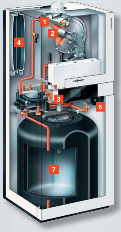
Vitodens 222-F mit emailiertem Ladespeicher
